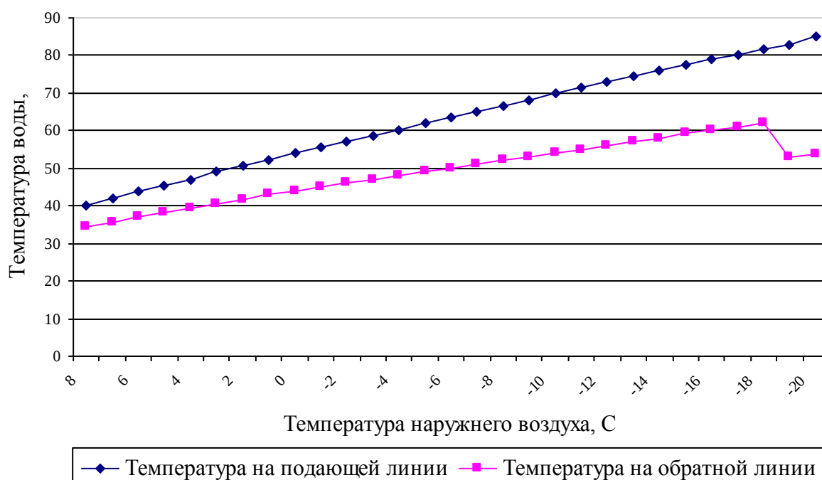
Рисунок 11.1.2.В – График зависимости температуры прямой и обратной сетевой воды от температуры наружного воздуха
